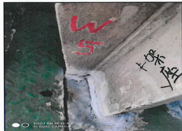
井架支座 1 号 W5 (应力测试前)
