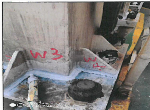
井架支座 1 号 W3 W4(应力测试前)
