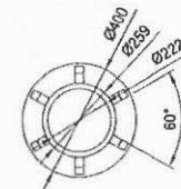
DETAIL B Scale: 1/10
