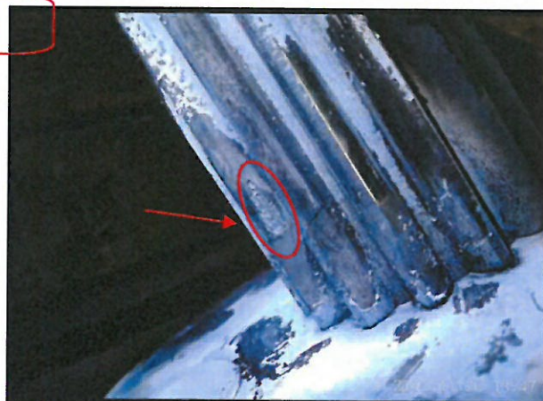
292HX29-00 3# (破损部分)
