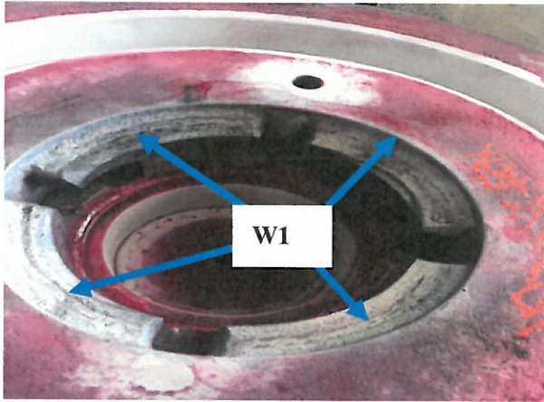
南海八号试压桩 W1
