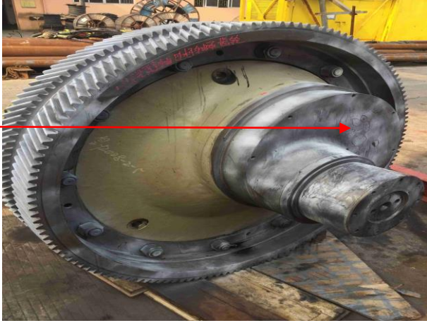
1 号泥浆泵主轴轴承齿轮
